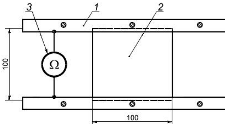
Рисунок 7 - Измерение электрического поверхностного сопротивления электропроводящей ткани
