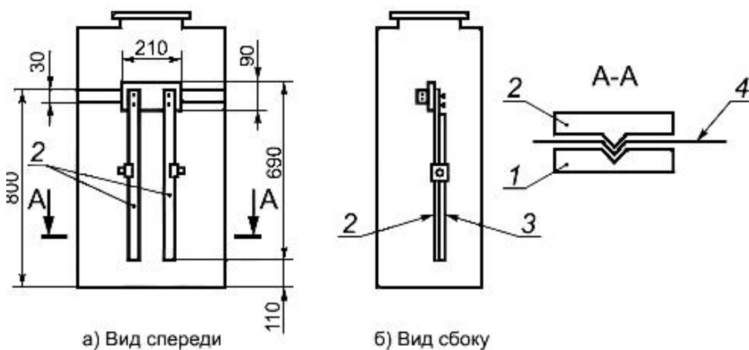
Рисунок 6 - Держатель испытуемого образца в испытательной камере
