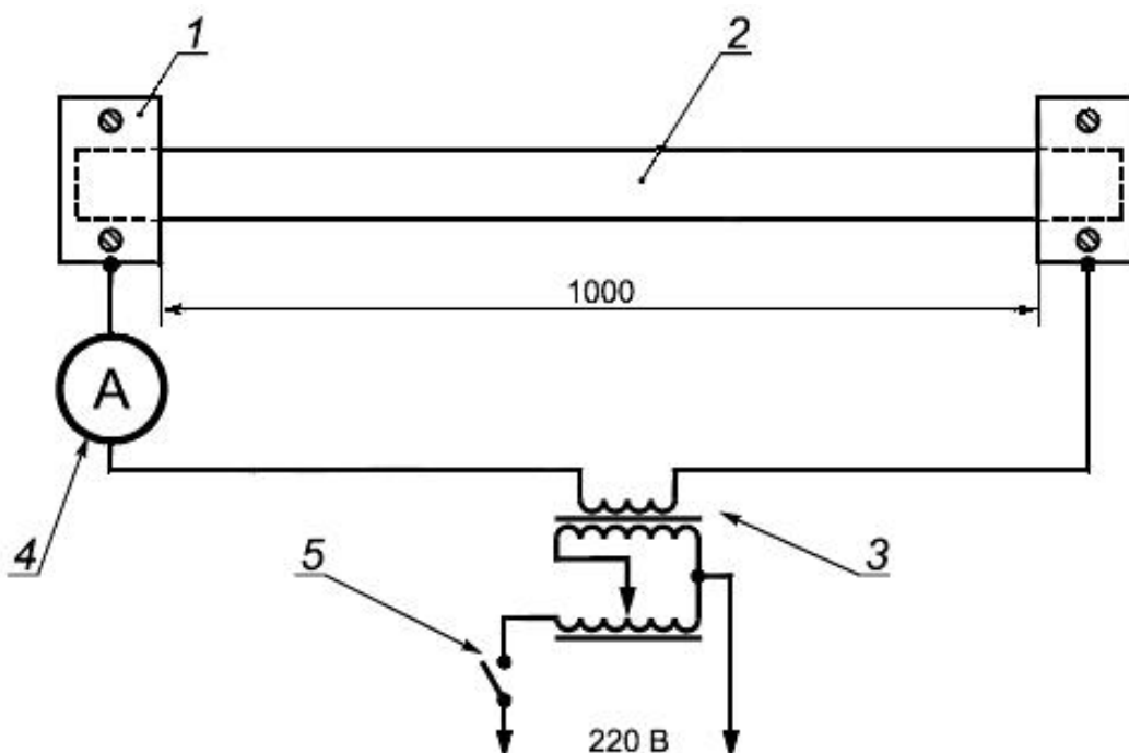
Рисунок 9 - Определение электрической проводимости электропроводящей ленты
