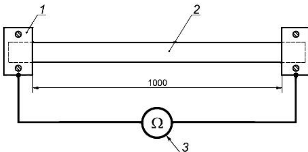
Рисунок 8 - Измерение электрического сопротивления электропроводящей ленты
