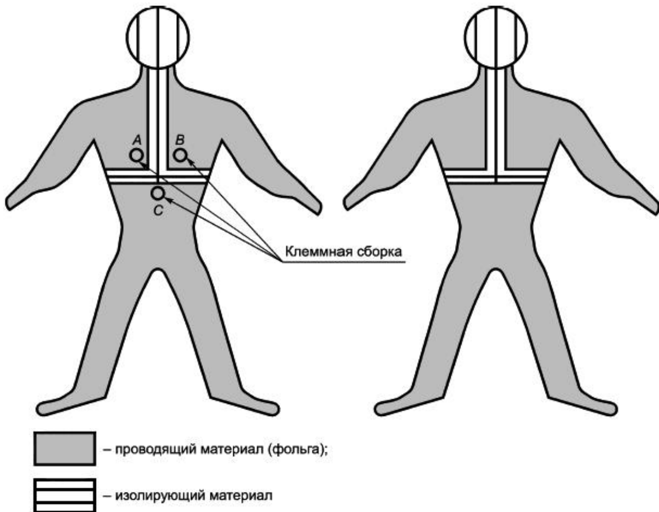
Рисунок 1 - Испытательный манекен, вид спереди и сзади
