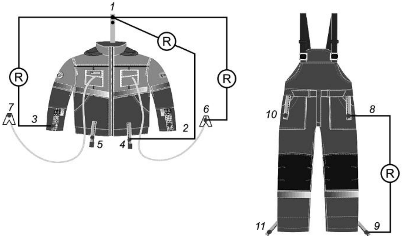
Рисунок 2 - Контактные выводы защитного комплекта
