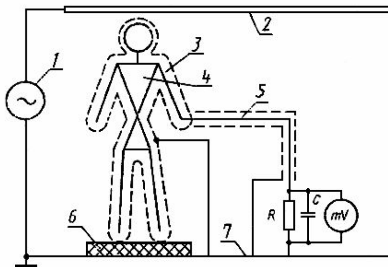
1 - источник высокого напряжения; 2 - электропроводящая пластина; 3 - комплект; 4 - электропроводящий манекен; 5 - провод; 6 - изолирующая подставка; 7 - заземляющая пластина
